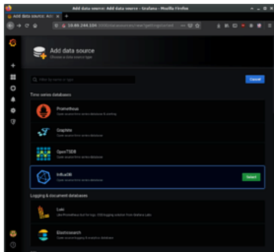
grafana_1960×888 79.3 KB
