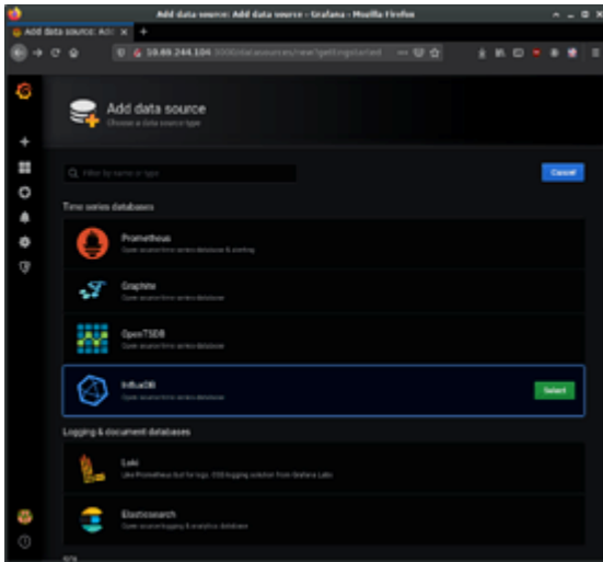
grafana_1960×888 79.3 KB
